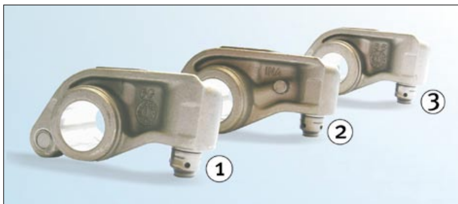
Foto. 1: Trzy różne zestawy dźwigienek
