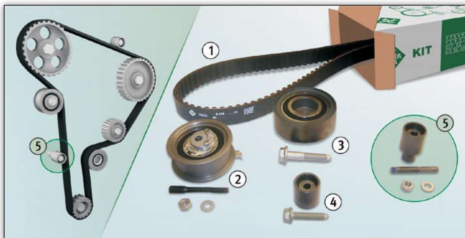
Foto 1: Schemat dla silnika 1.9 TDI/SDI oraz zawartość opakowania zestawu KIT 530 0361 10 / 530 0082 10
