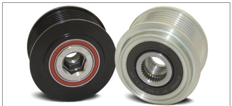
Foto2: Wolne koło alternatora 535 0229 10
